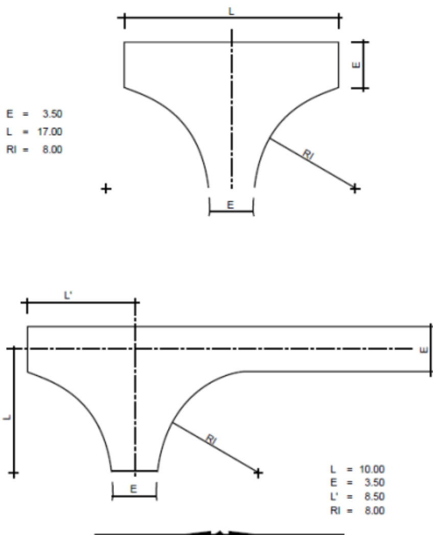
COTES MINIMALES DES AIRES DE MANŒUVRE pour bennes tasseuses de collecte d'ordures ménagères dans une voie en impasse.
